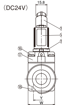
(DC24V)
